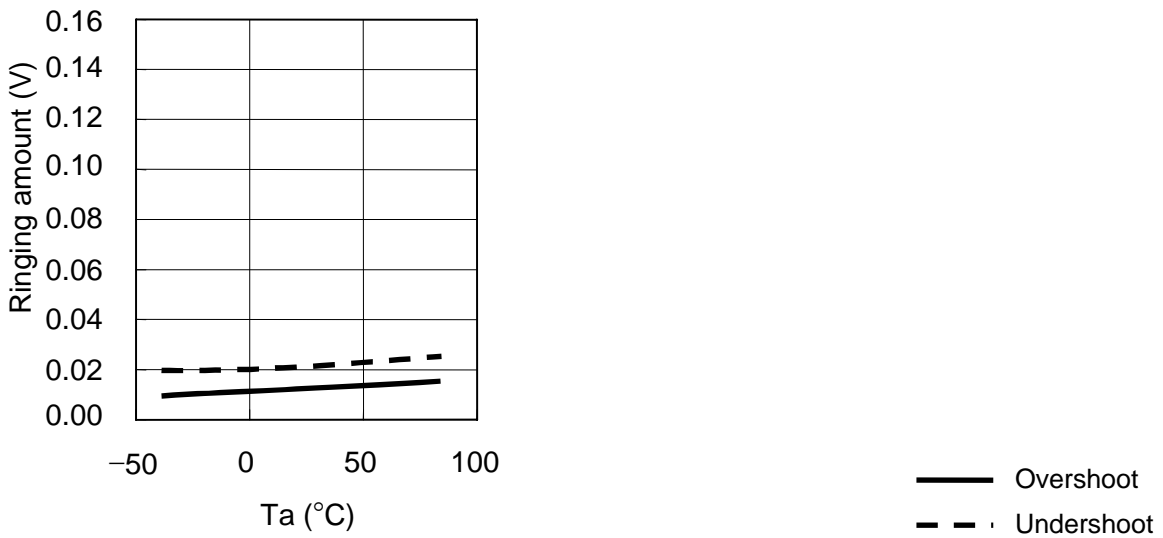
(3) VCH pin
